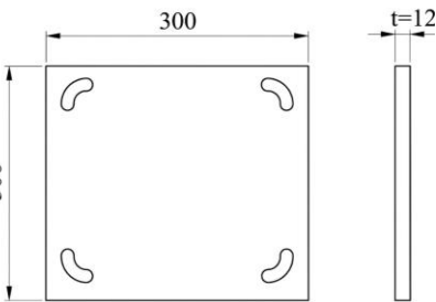
FLANŞ 300x300 (t=12 mm)
