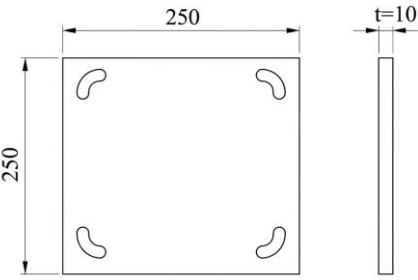
FLANŞ 250x250 (t=10 mm)
