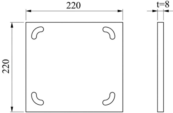
J ANKRAJ DETAYI (M12)
