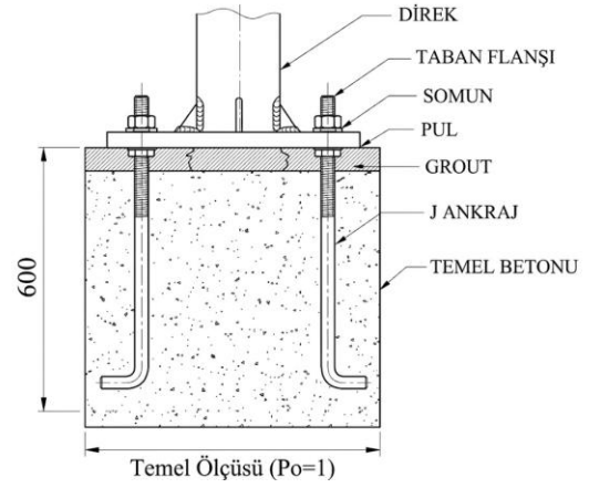
MONTAJ VE TEMEL DETAYI (ÖRNEK)
