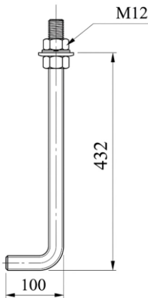
J ANKRAJ DETAYI (M12)
