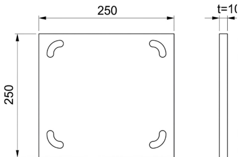
FLANGE 250x250 (t=10 mm)
