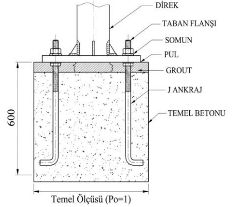
MONTAJ VE TEMEL DETAYI (ÖRNEK)
