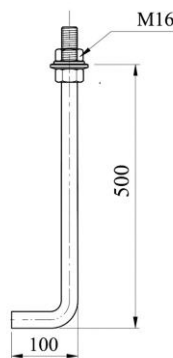
J ANKRAJ DETAYI (M16)
