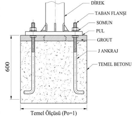
MONTAJ VE TEMEL DETAYI (ÖRNEK)
