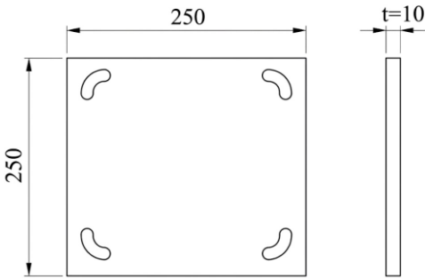
FLANŞ 250x250 (t=10 mm)
