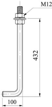
J ANKRAJ DETAYI (M12)
