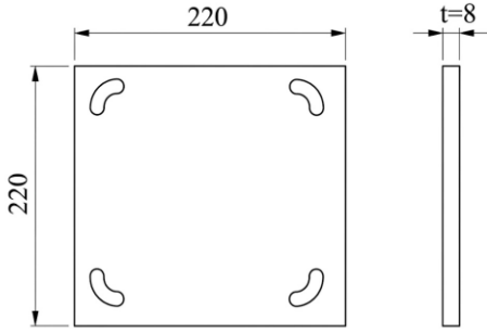
J ANKRAJ DETAYI (M12)
