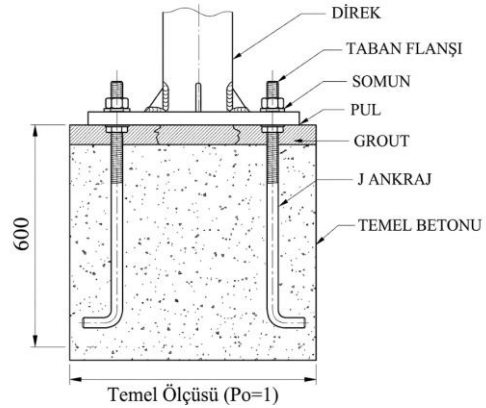
MONTAJ VE TEMEL DETAYI (ÖRNEK)
